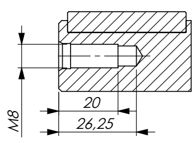
SEZIONE D-D
