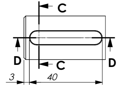
DETTAGLIO B
