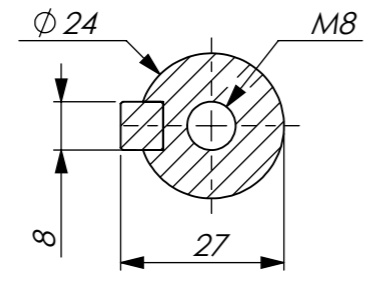
SEZIONE C-C
